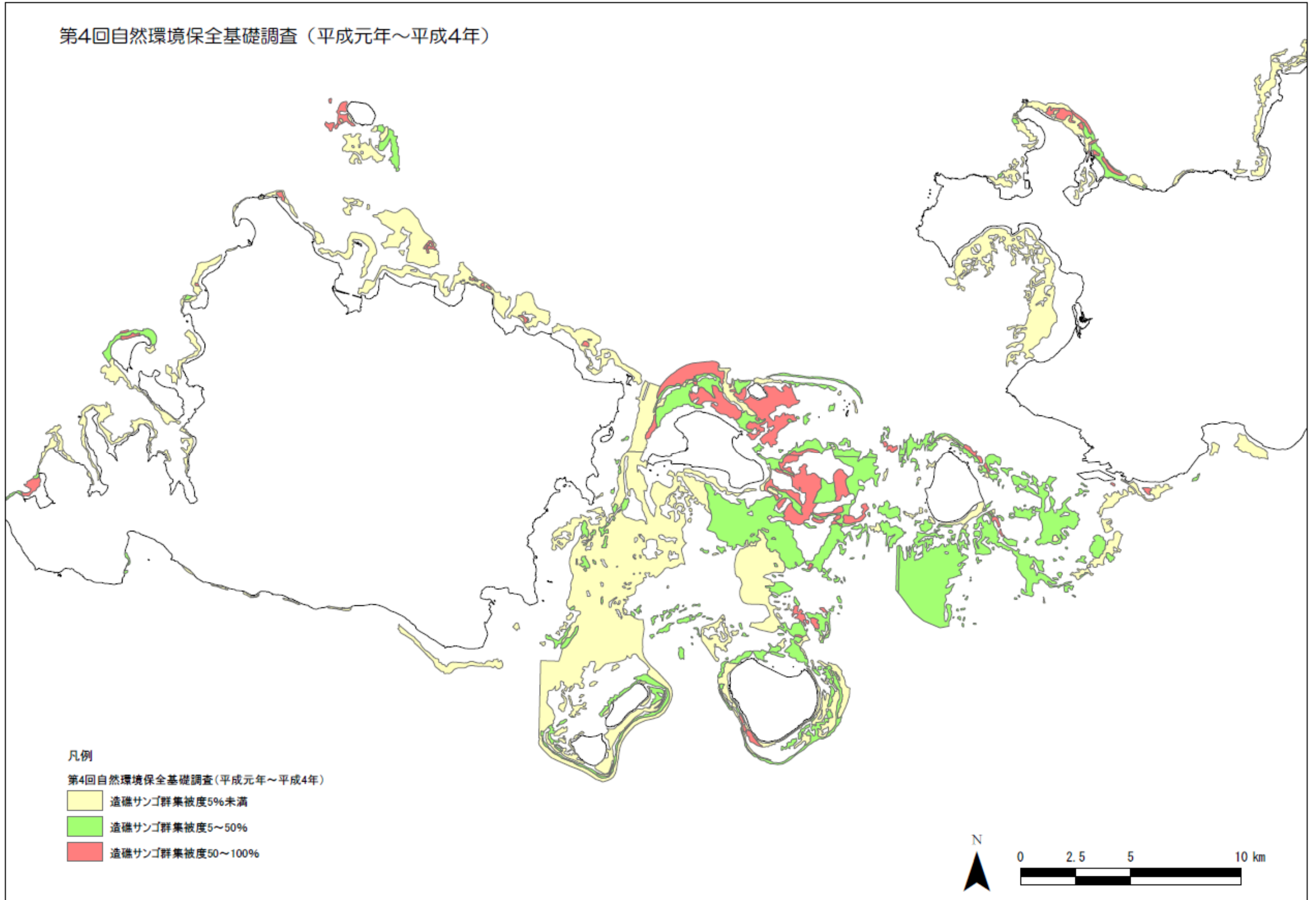
図 2.3.7-1(1) 造礁サンゴ群集被度分布（第4回自然環境保全基礎調査）〈1989-1992〉
