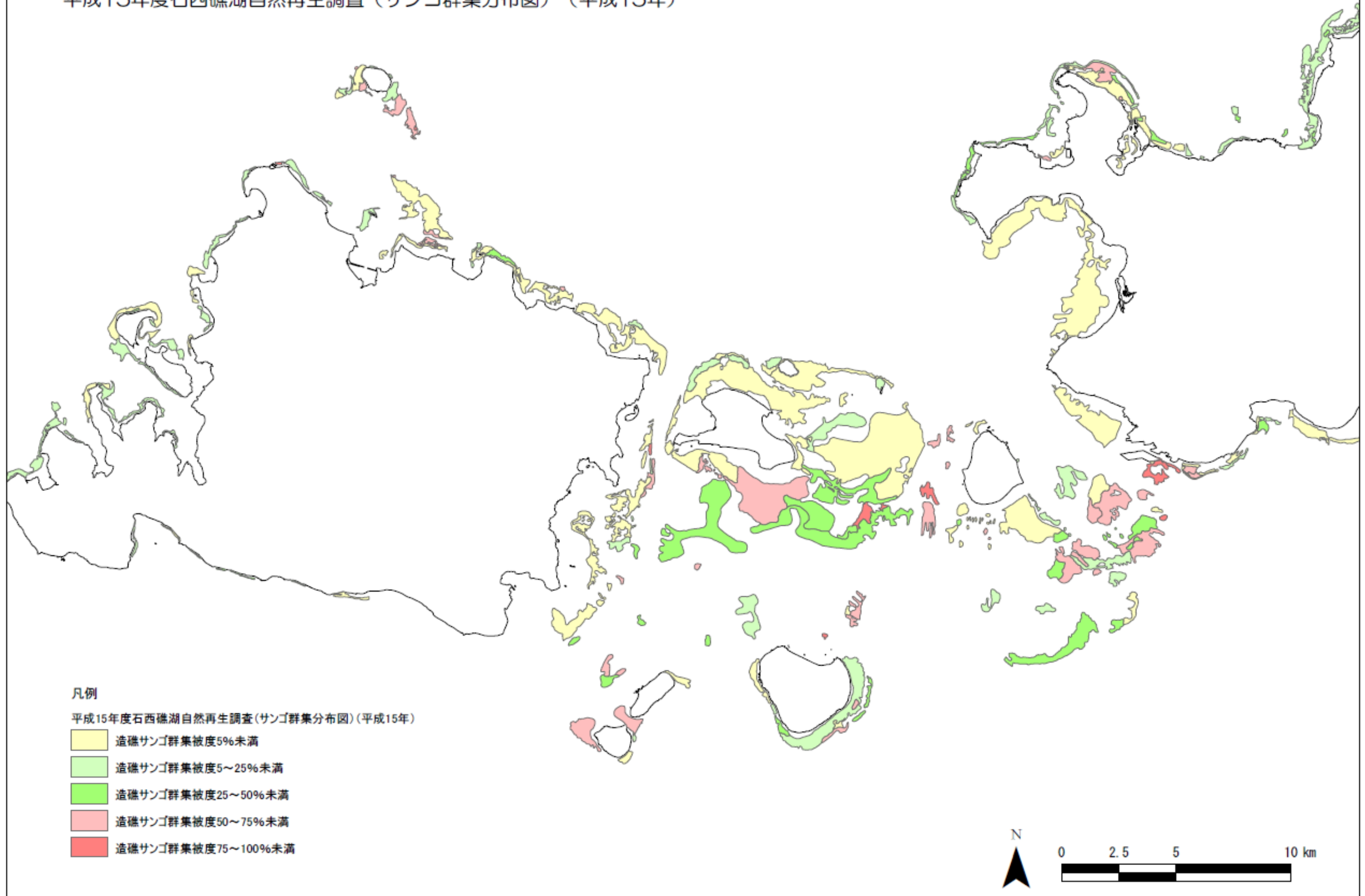
図 2.3.7-1(2) 造礁サンゴ群集被度分布(平成15年度石西礁湖自然再生調査)<2003年>
