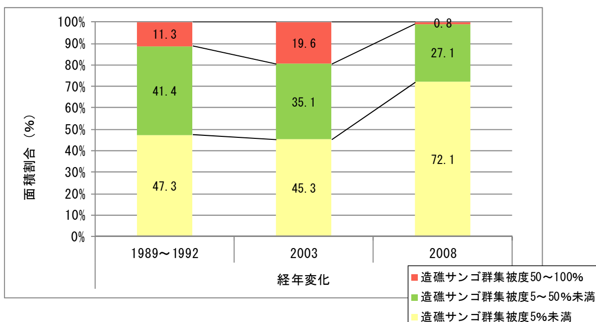
図 2.3.7-3 造礁サンゴ群集被度区分毎の面積割合変化
