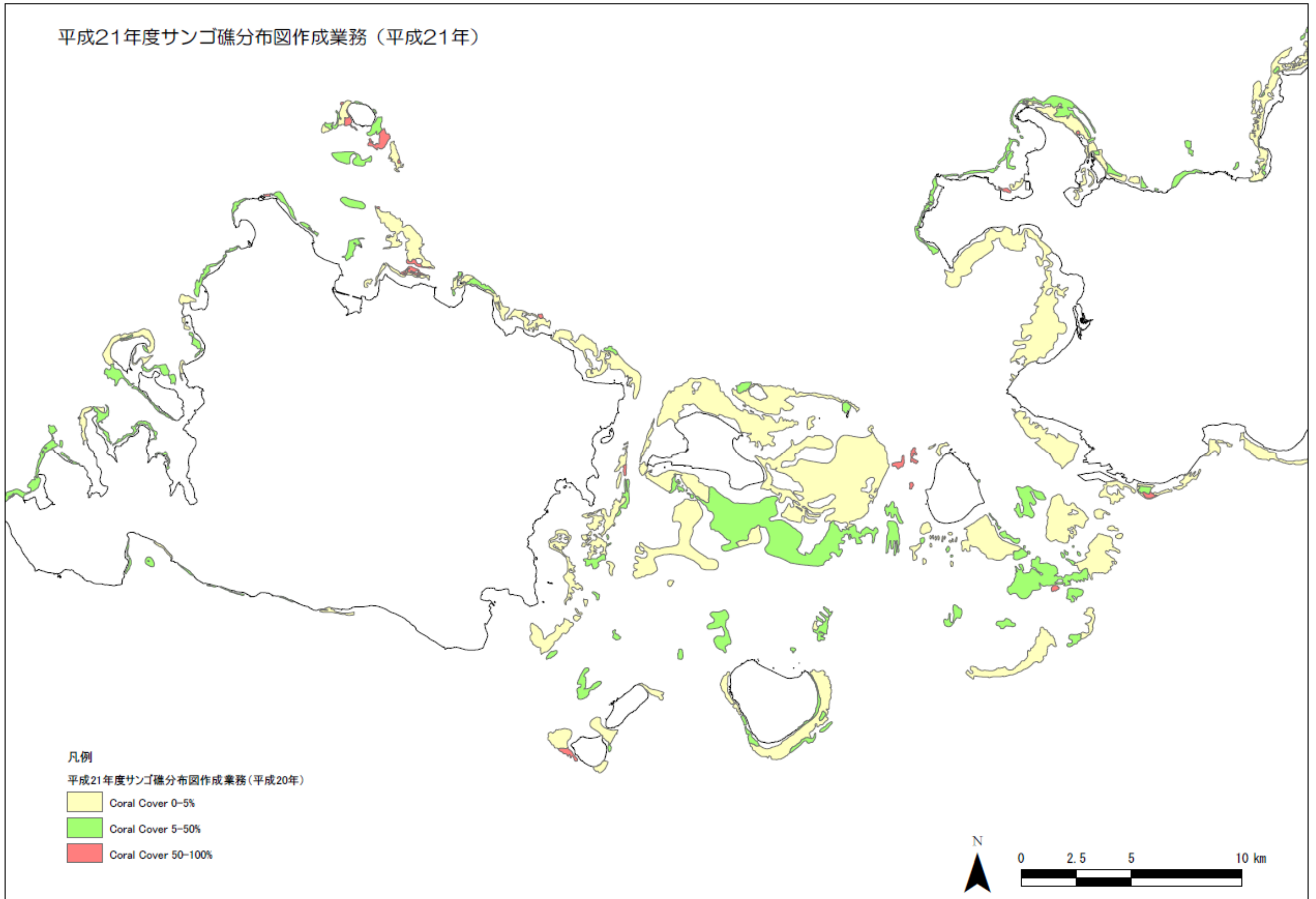
図 2.3.7-1 (3) 造礁サンゴ群集被度分布（平成 21 年度サンゴ礁分布作成業務）〈2008 年〉
