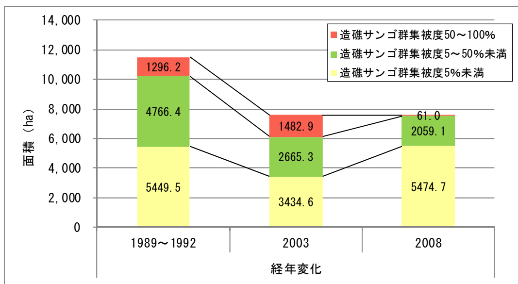
図 2.3.7-2 造礁サンゴ群集被度区分毎の面積変化
